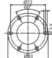
Flangia con fori di fissaggio FSB/25
