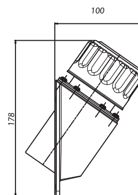
Flangia con fori di fissaggio FSB/25
