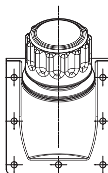
Flangia con fori di fissaggio FSB/05
